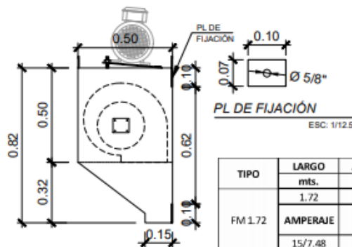
ELEVACIÓN "B" CORTINA DE AIRE ESC: 1/25 ③
