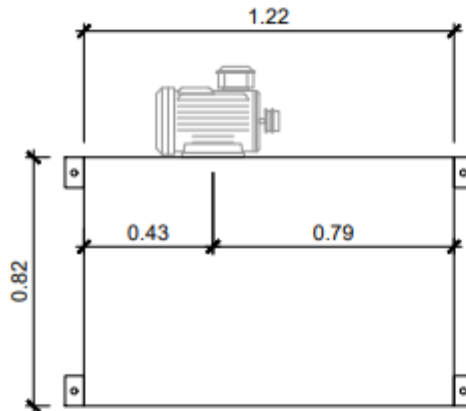
ELEVACIÓN "A" CORTINA DE AIRE ESC: 1/25 ②
