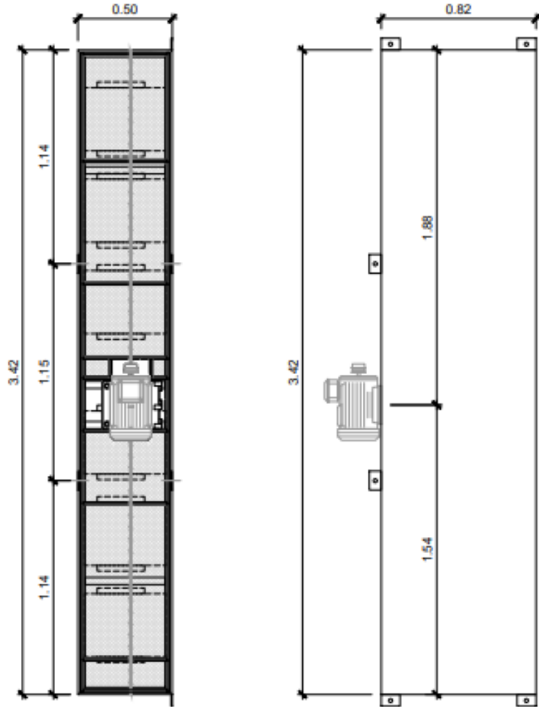
PLANTA CORTINA DE AIRE ESC: 1/25 ①
