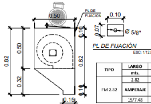
ELEVACIÓN "B" CORTINA DE AIRE ESC. 1/25 ③
