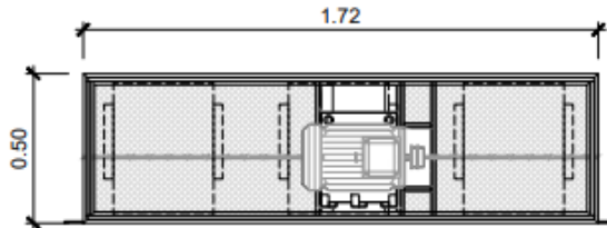
PLANTA CORTINA DE AIRE ESC: 1/25 ①
