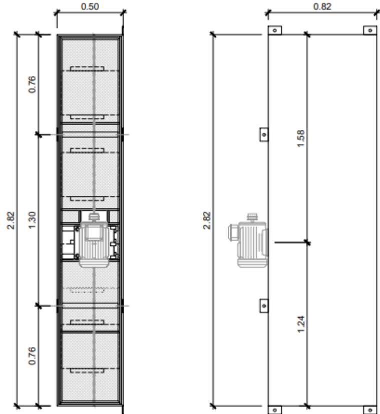
PLANTA CORTINA DE AIRE ESC. 1/25 ①
