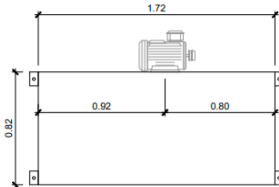
ELEVACIÓN "A" CORTINA DE AIRE ESC: 1/25 ②
