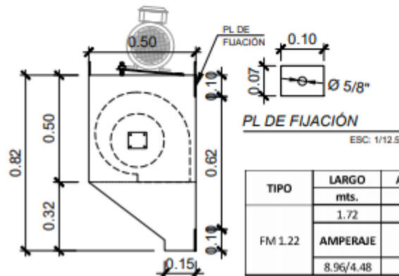
ELEVACIÓN "A" CORTINA DE AIRE ESC: 1/25 ②
