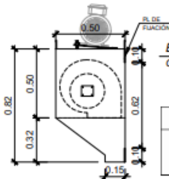
PLANTA CORTINA DE AIRE ESC: 1/25 ①
