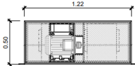
PLANTA CORTINA DE AIRE ESC: 1/25 ①
